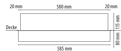
UV-C-Aufbaugerät Cloud
